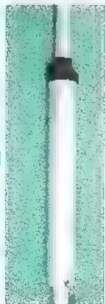
Commerciële trap, de buitenste buis beschermt de spoel en dient tevens zelf als condensator. Aan de bovenkant afgesloten met een sluitende kap.
